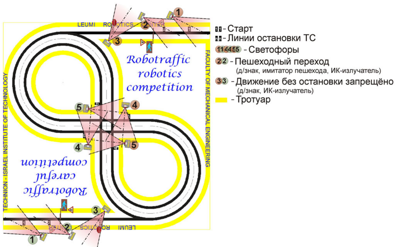
Рис. Оснастка поля категории А - Модель "городского уличного движения" (РобоТраффик - 2022)
